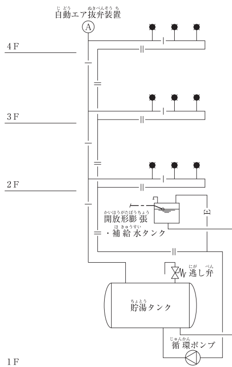
(8) 給湯設備系統図
