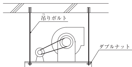
(7) 送風機（呼び番号2未満）吊り要領図
