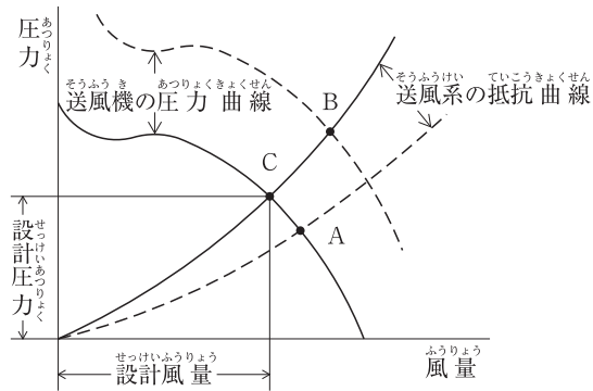
図-2 特性曲線
