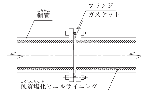
(7) 水道用硬質塩化ビニルライニング鋼管フランジ接合断面図
